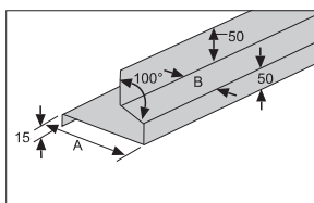
Надоконная планка
