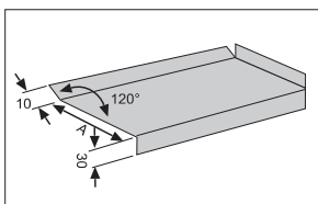
Подоконная планка
